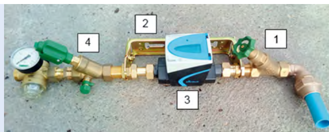
1. Absperrarmatur Versorgerseite, 2. Zählerbügel nach DVGW DIN 1988-200, 3. Wasserzähler, 4. KFR-Ventil (Absperrarmatur mit Rückflussverhinderer) Hausseite Foto: Fa. Sensus
