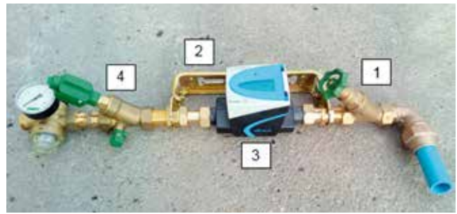
1. Absperrarmatur Versorgerseite, 2. Zählerbügel nach DVGW DIN 1988-200, 3. Wasserzähler, 4. KFR-Ventil (Absperrarmatur mit Rückflussverhinderer) Hausseite Foto: Fa. Sensus
